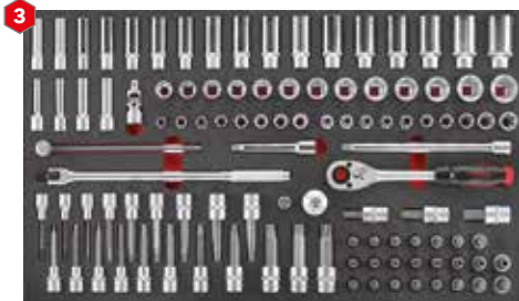
FOR F41062 doppenset 1/2" 106dlg, jeu de douilles 106pcs
